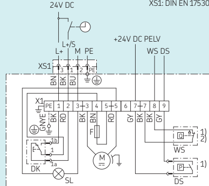
Versione D MKU2-12BC11000+924
