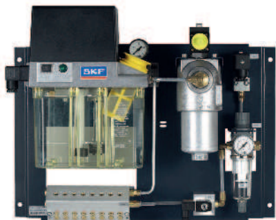
Unità di lubrificazione olio+aria SKF OLA8-1B6BB... (Configurazione completa)
