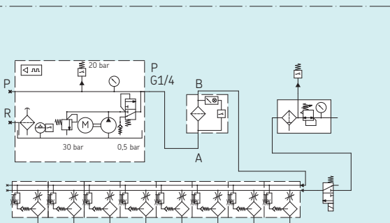
Unità di lubrificazione olio+aria con unità di controllo
