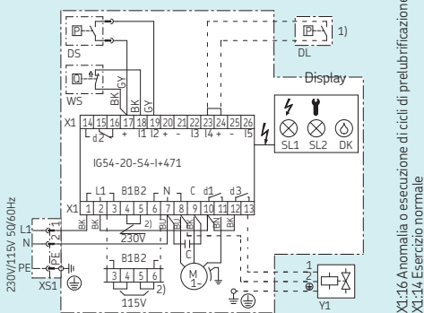
Versione B / C MKL2-12FC11000+428 /+429
