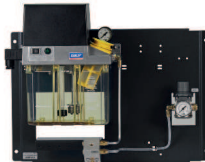
Unità di lubrificazione olio+aria SKF OLA1-1B0XA... (Configurazione minima)
