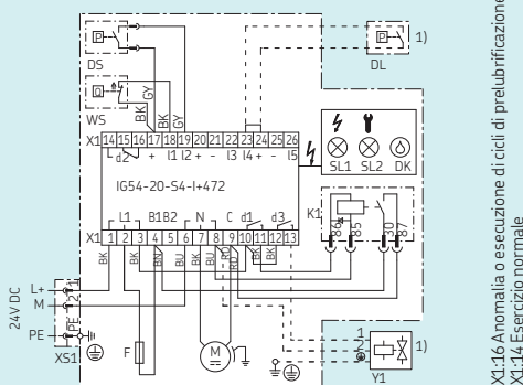
Versione A MKL2-12FC11000+924
