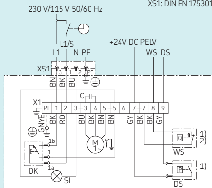
Versione E / F MKU2-12BC11000+428 /+429
